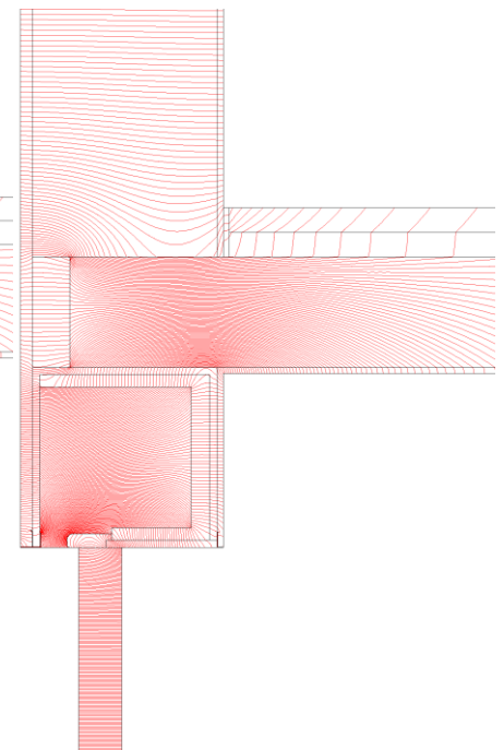
mit 20 mm ROLAFLEX®
